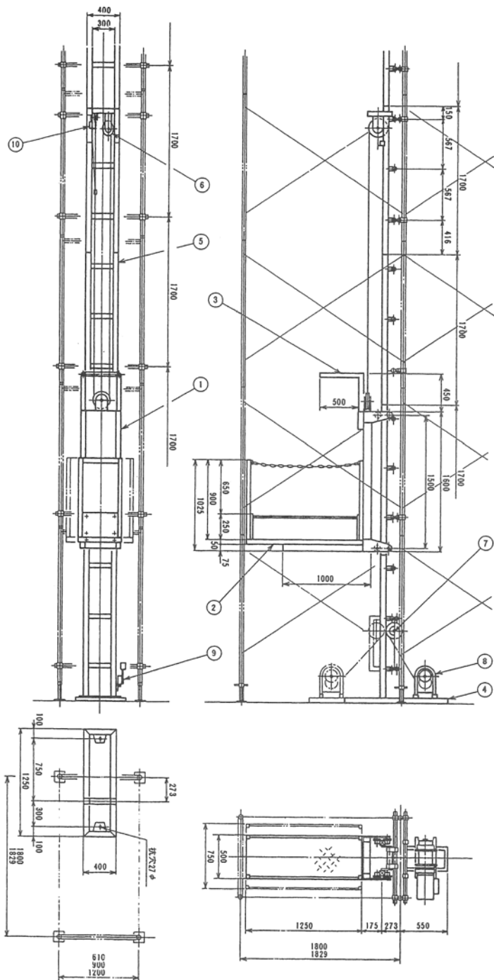
A-A 矢視図
