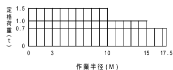
性能線図
