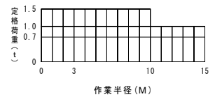
性能線図
