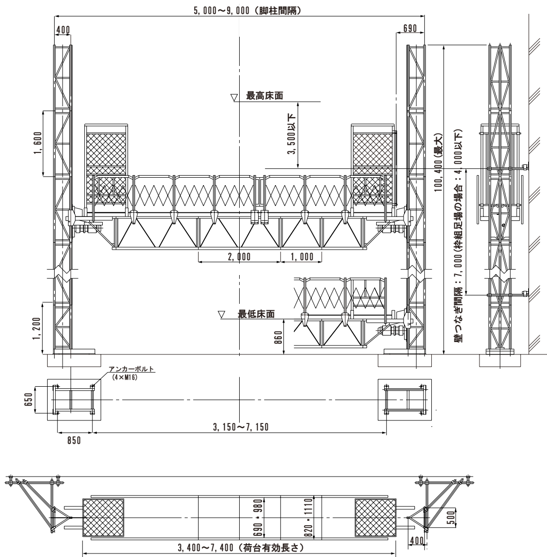
【全体仕様図】
