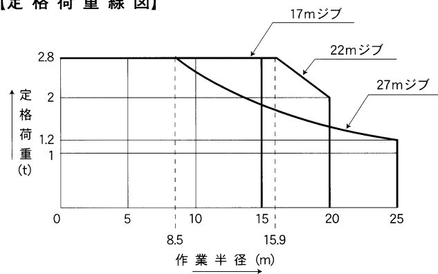
【定格荷重線図】
